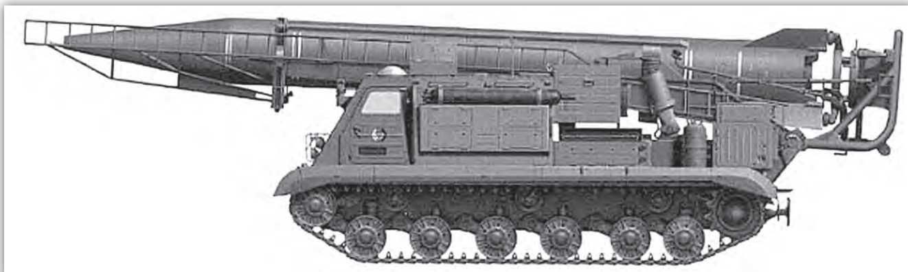
Самоходная пусковая установка ракеты Р-11М
